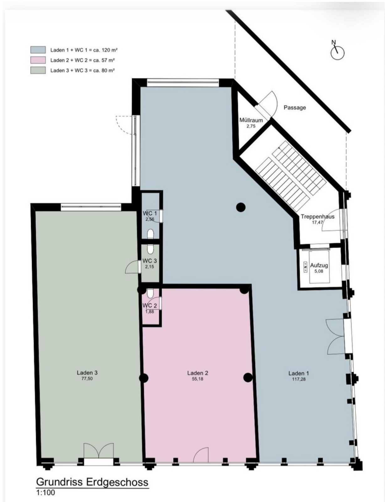
Grundriss - Laden 3
