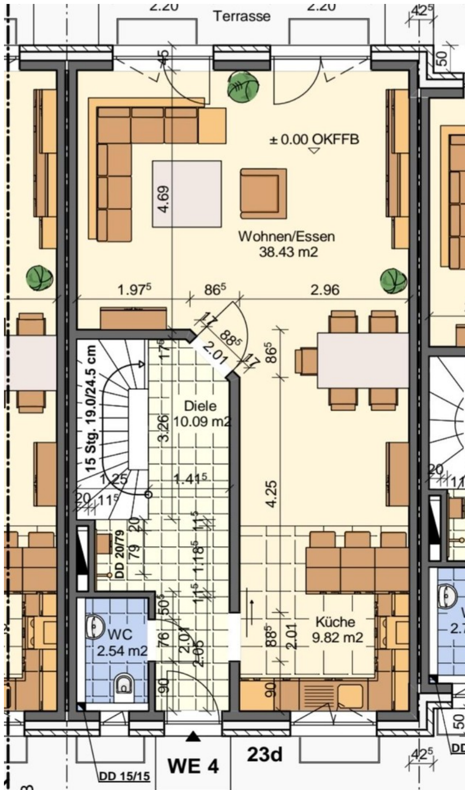
EG Grundriss
