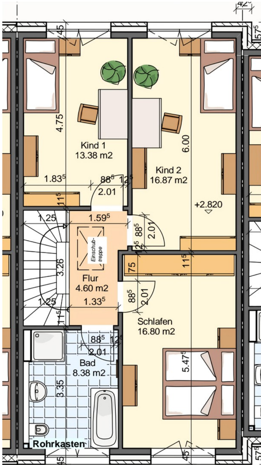
OG Grundriss
