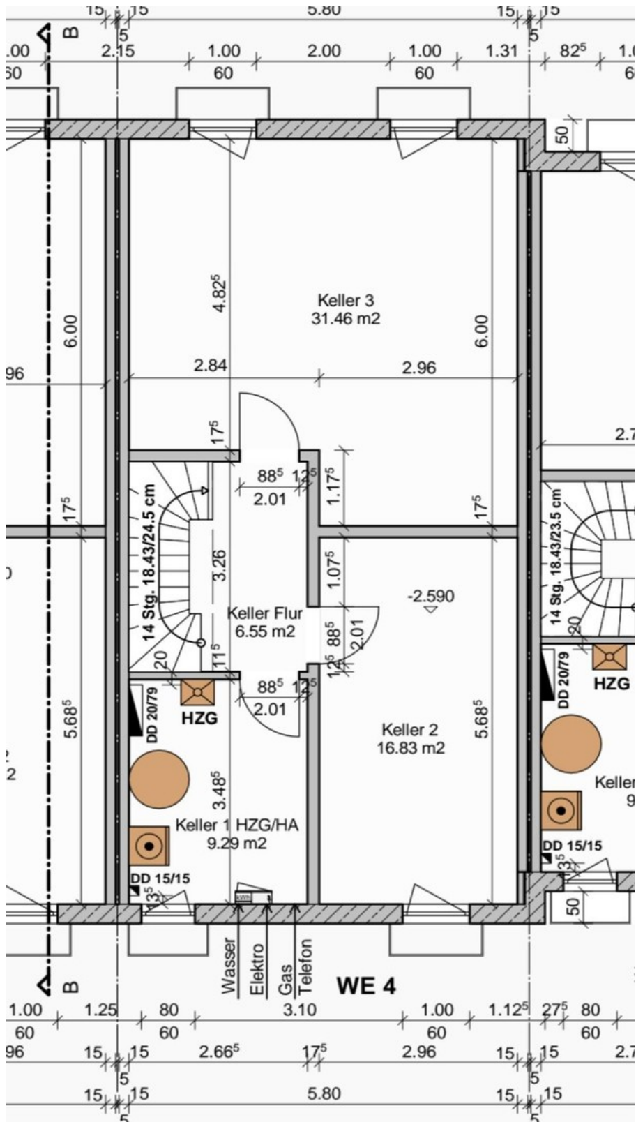
Keller Grundriss
