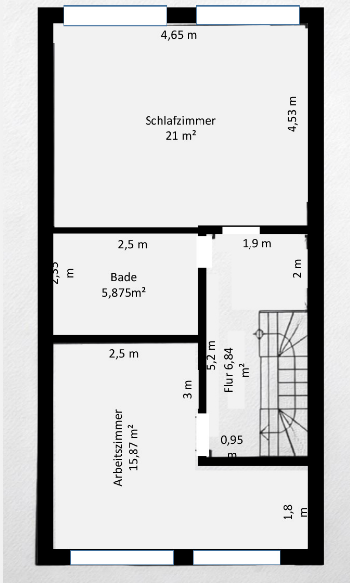
Obergeschoss 49,58 m 2
