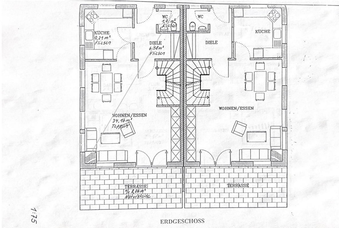
Erdgeschoss
