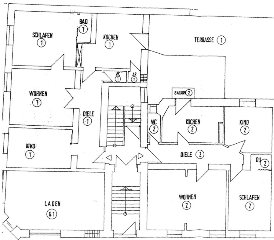
Grundriss Wohnung 1
