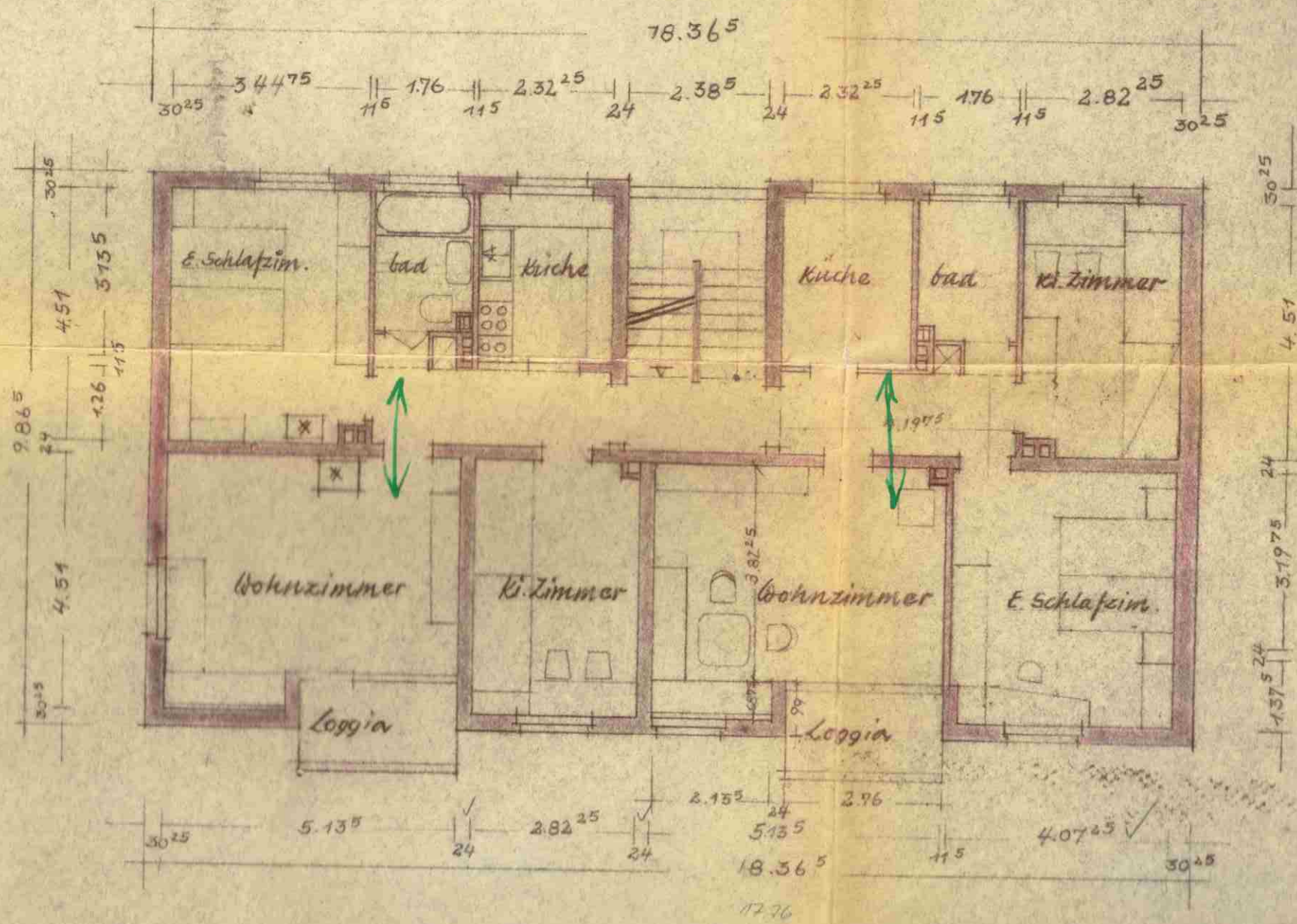
ERDGESCHOSS 1-2 OBERGESCHOSS
