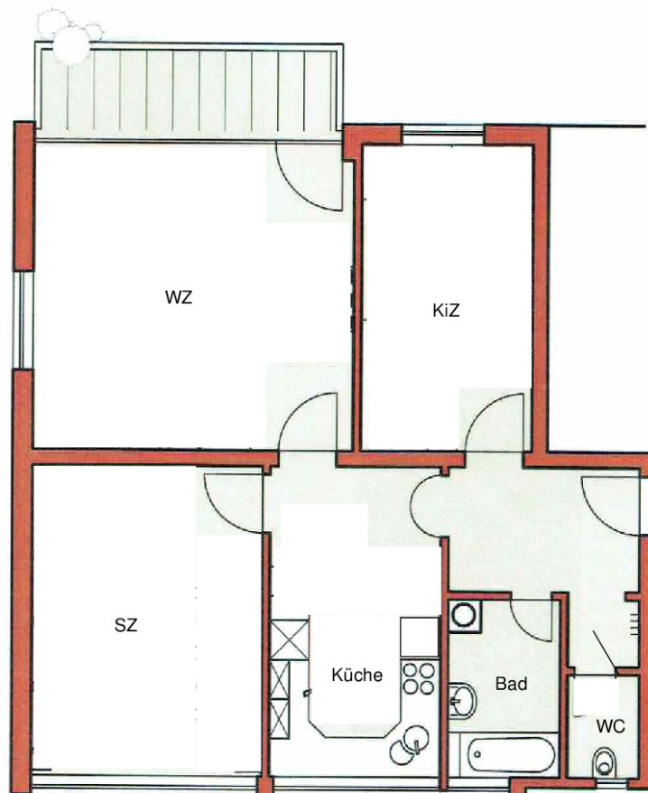
GRUNDRISS
