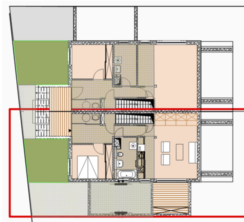
Untergeschoß
