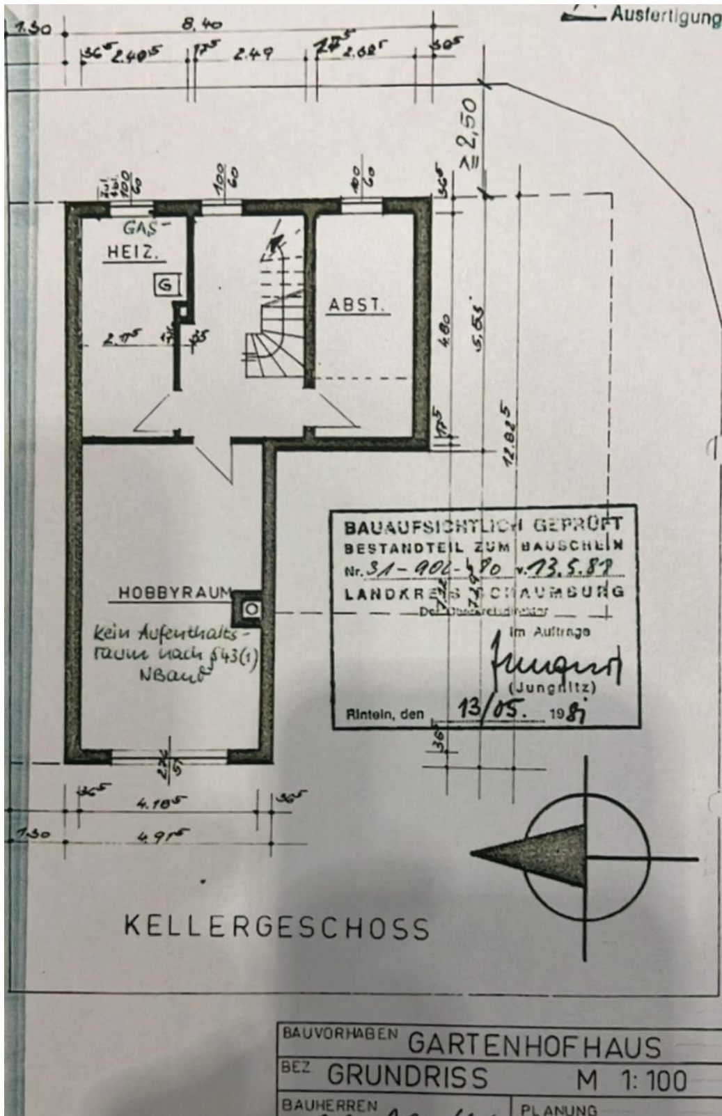
Grundriss Keller
