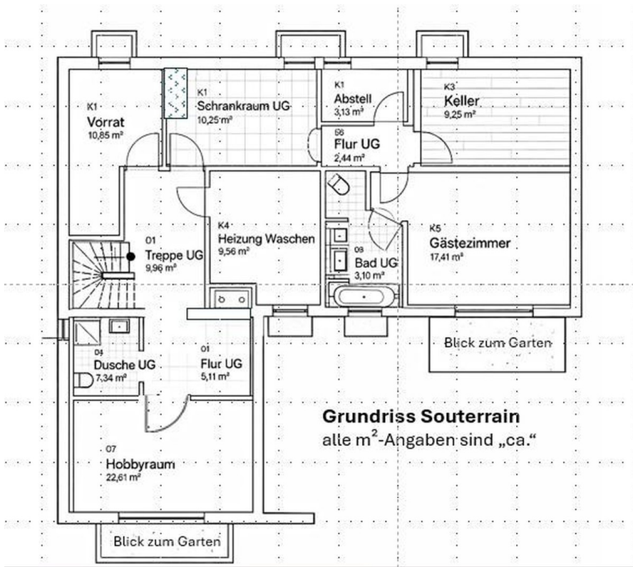
Grundriss Souterrain
