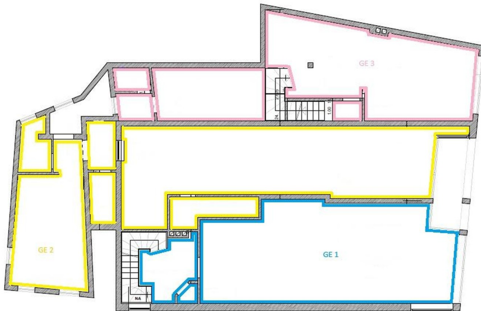
Grundriss EG
