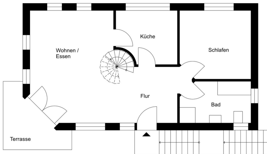
ERDGESCHOSS
