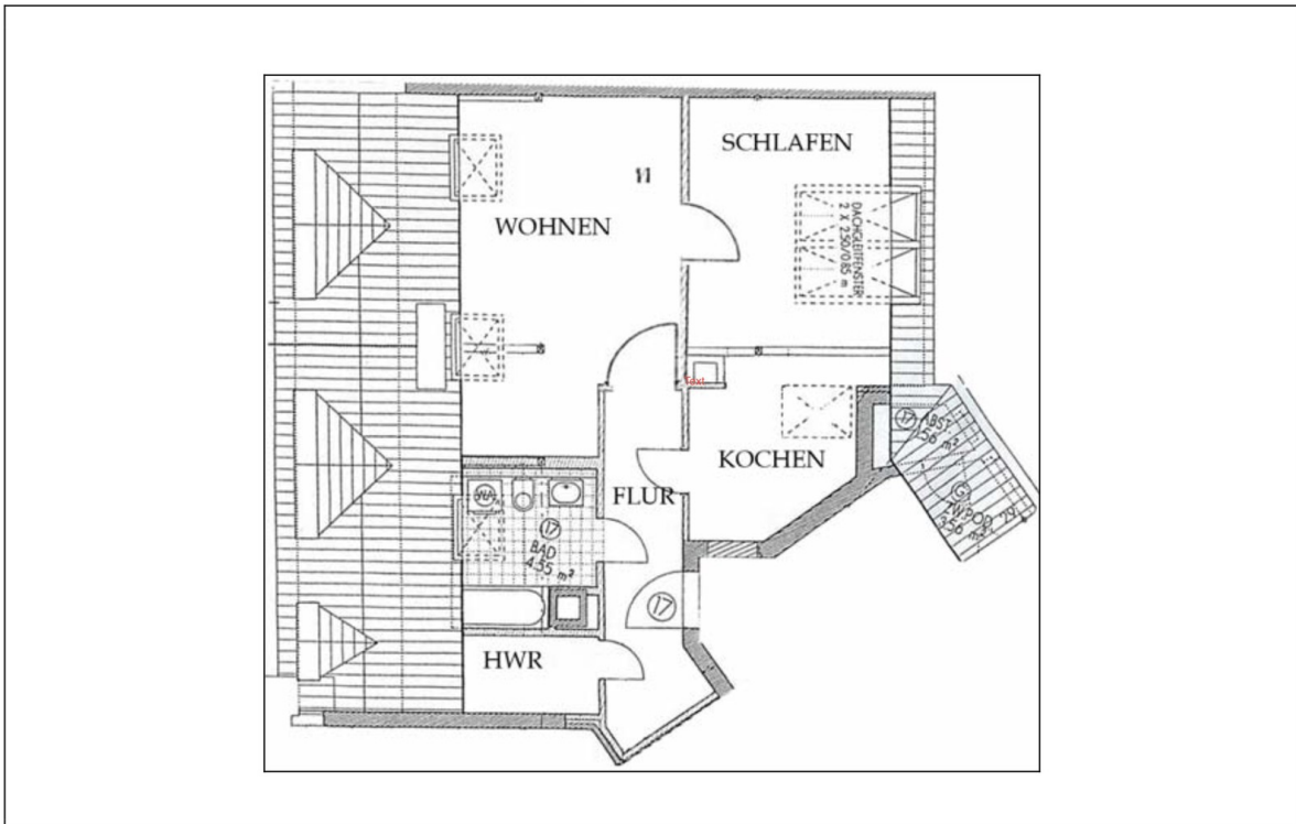
Grundrisskizze
