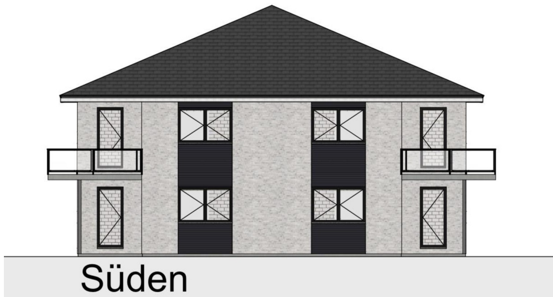
Ansicht Süden
