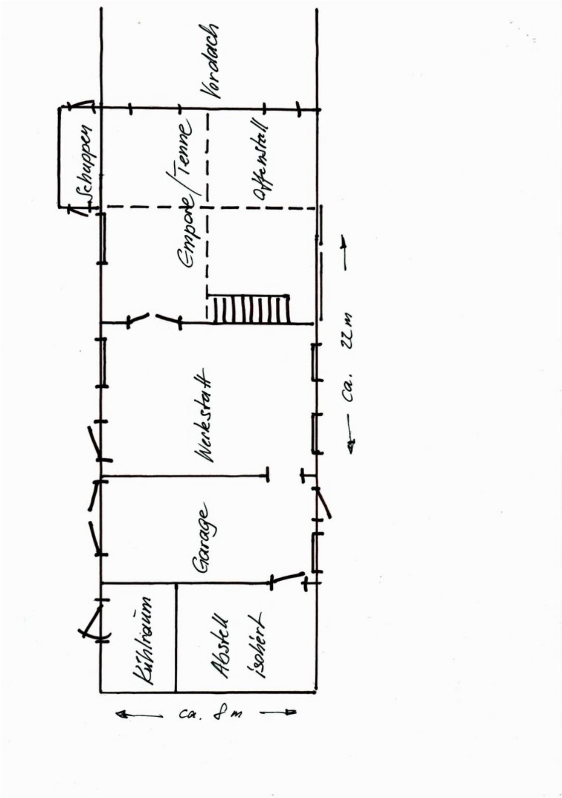
Grundriss Remise
