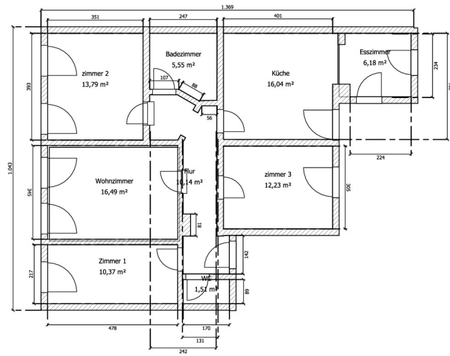
Wfg. 5 Etage 2 Wohnfläche : 92,30 qm
