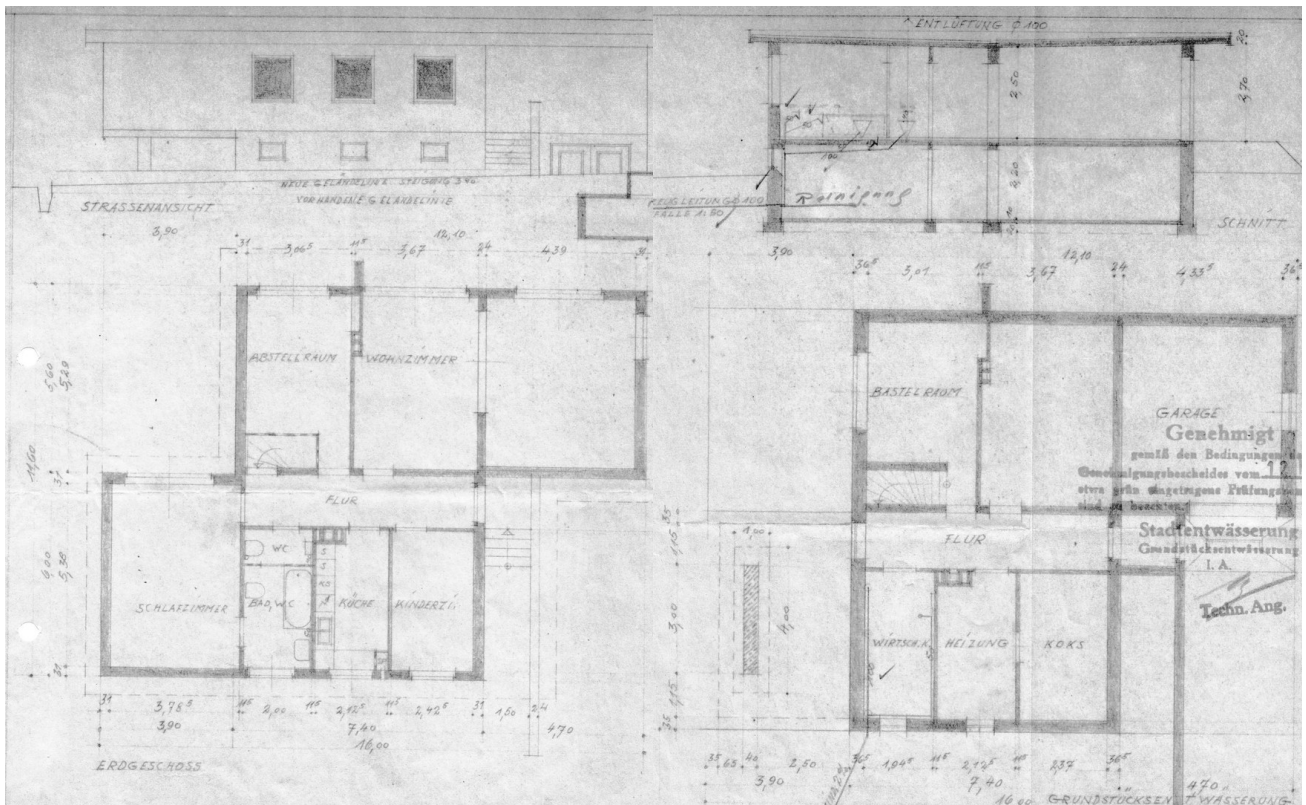
Grundriss/Ansicht 1
