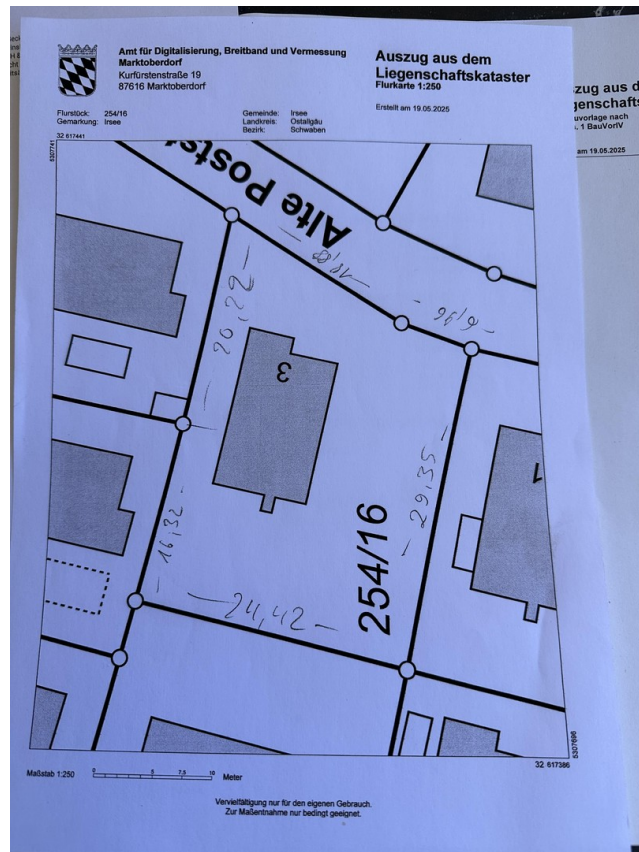
Plan mit Bemaßungen
