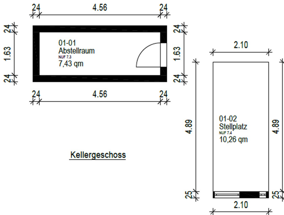
Grundriss Keller/TG-Stellplatz
