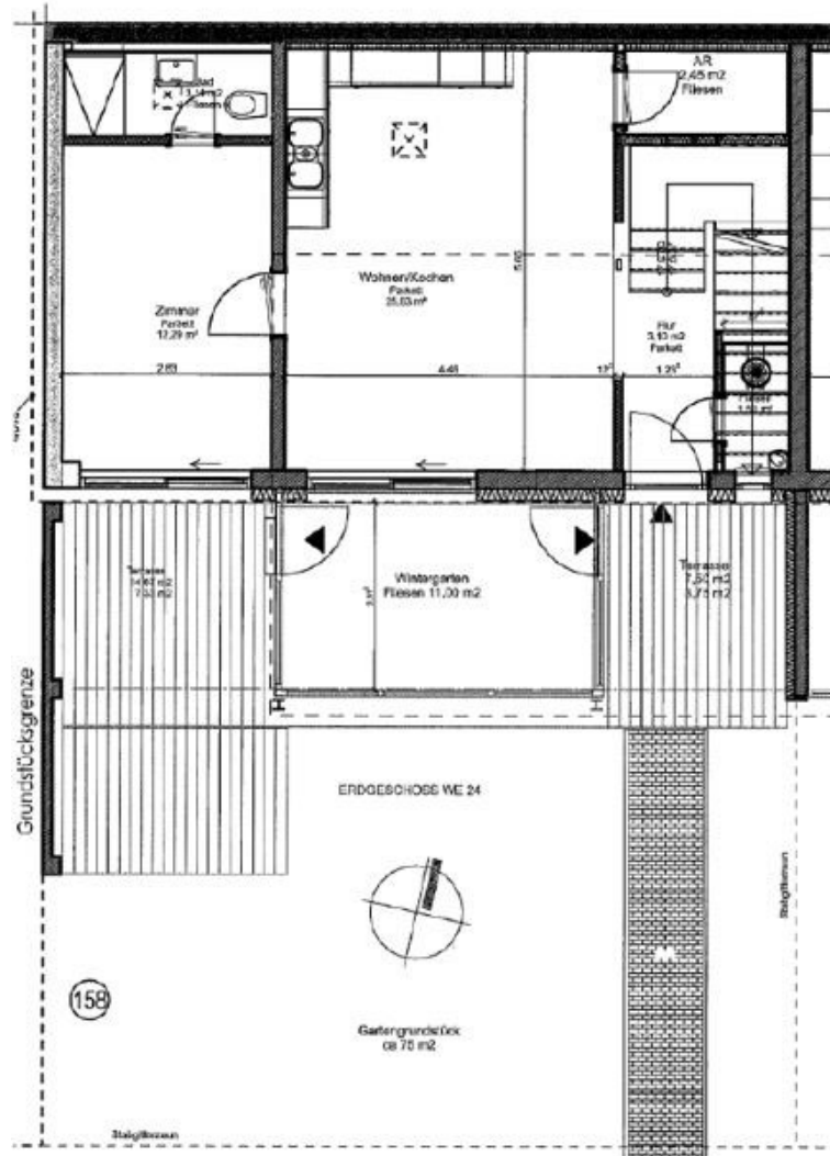
Gartengeschoss
