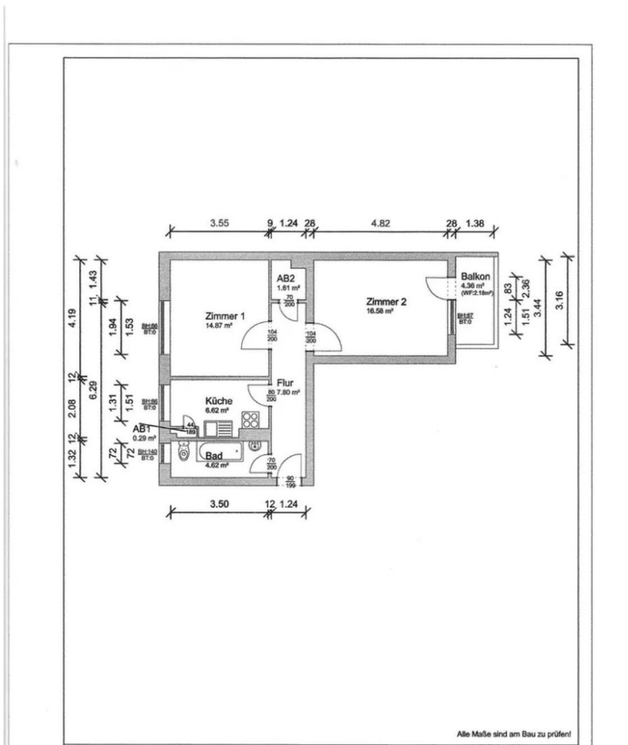
Grundriss
