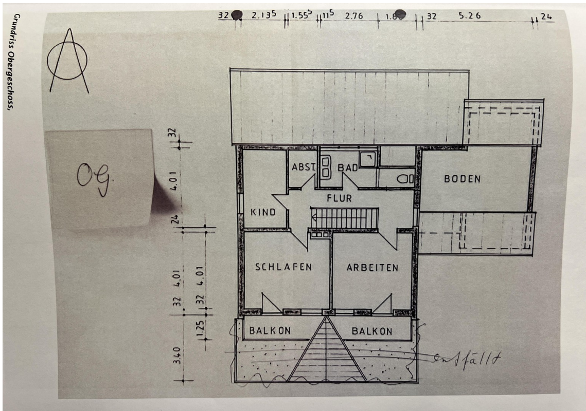
Grundriss OG
