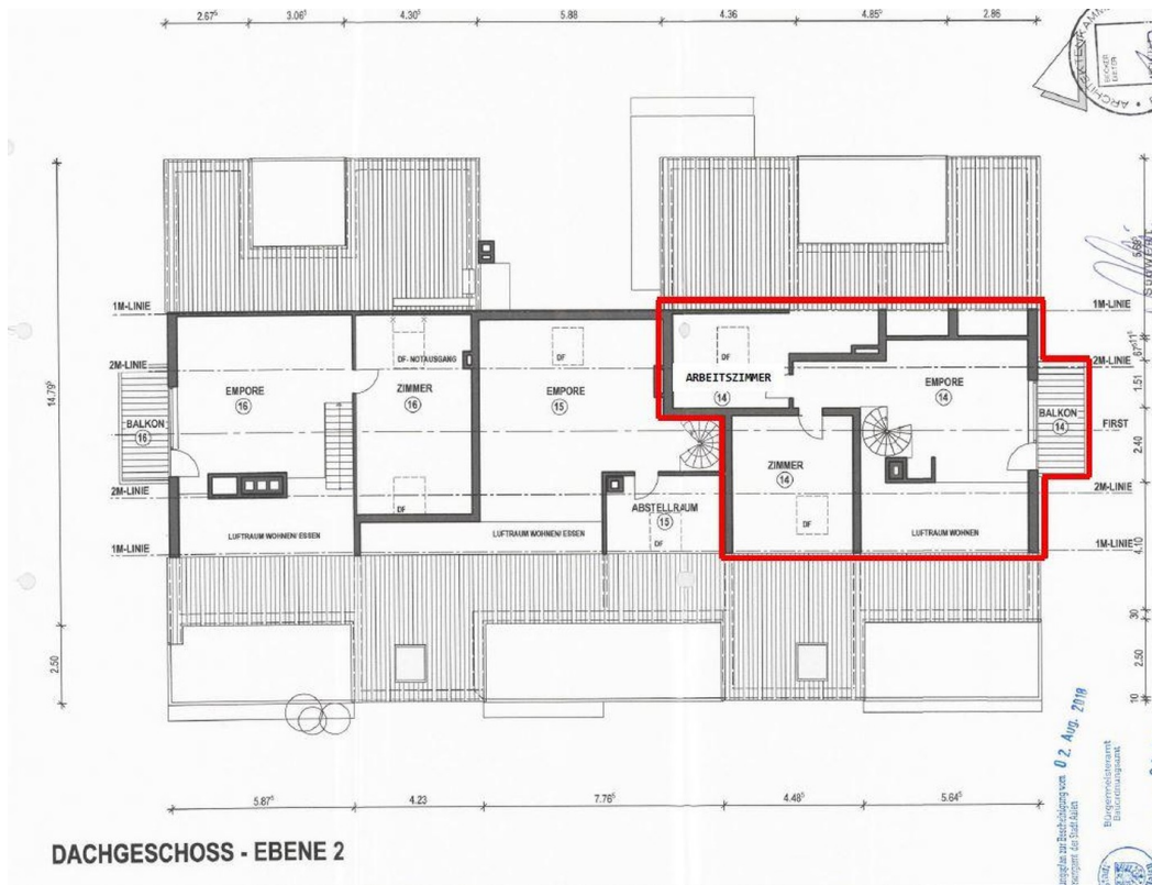
Grundriss DG2
