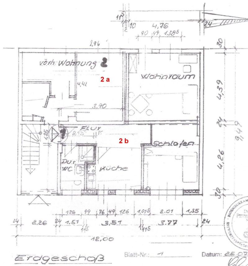
Erdgeschoss
