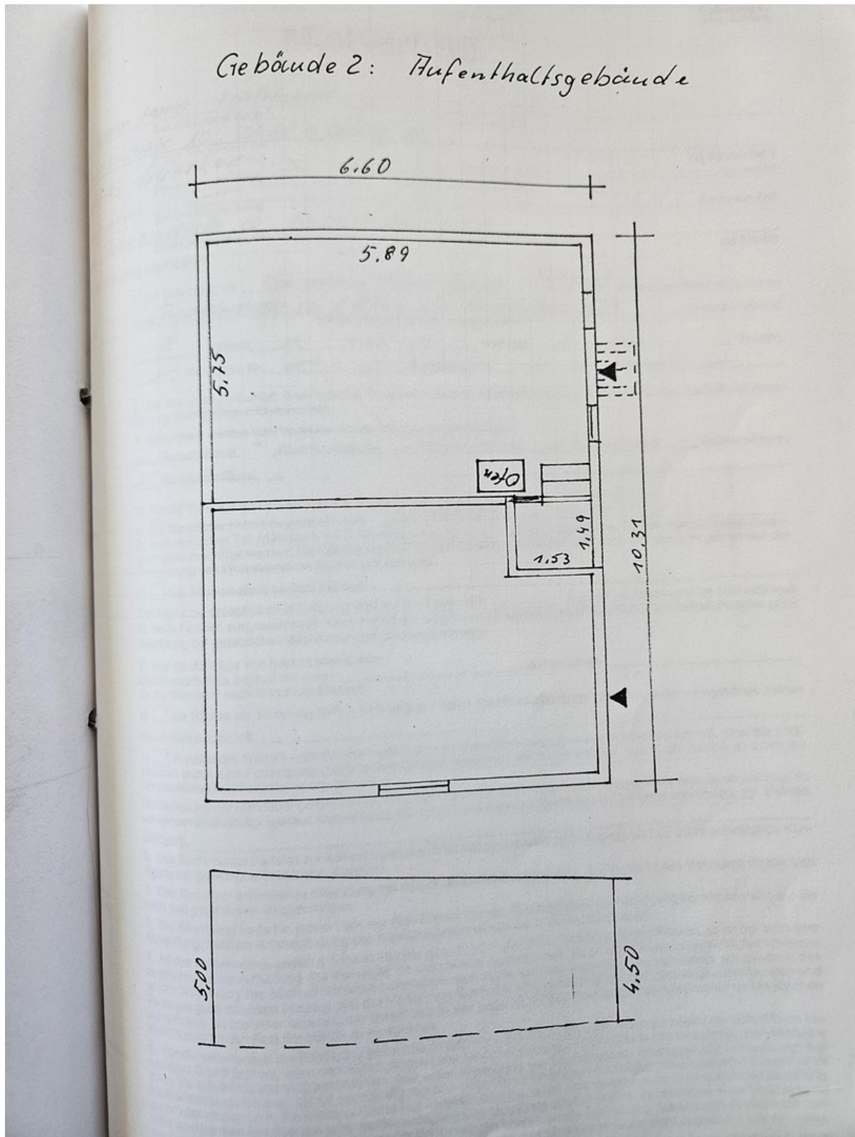
Grundriss Nebengebäude
