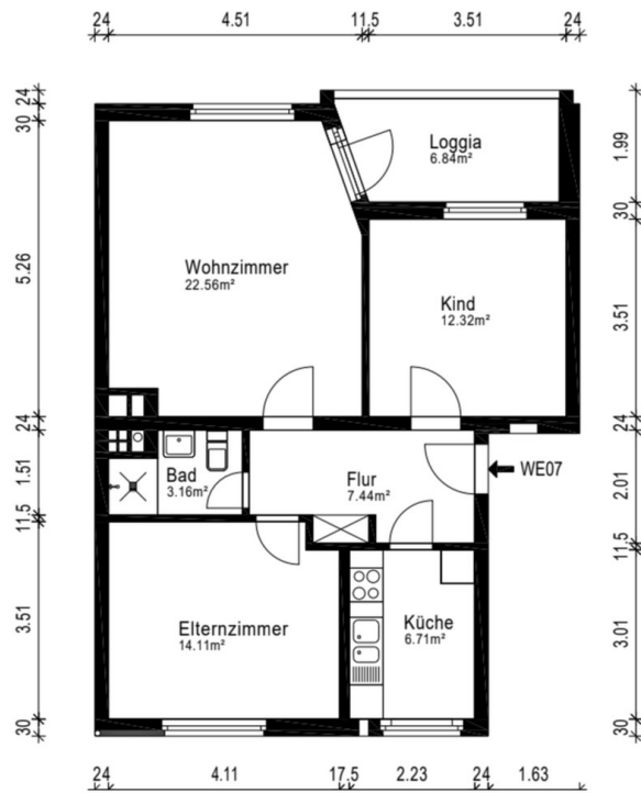
Grundriss
