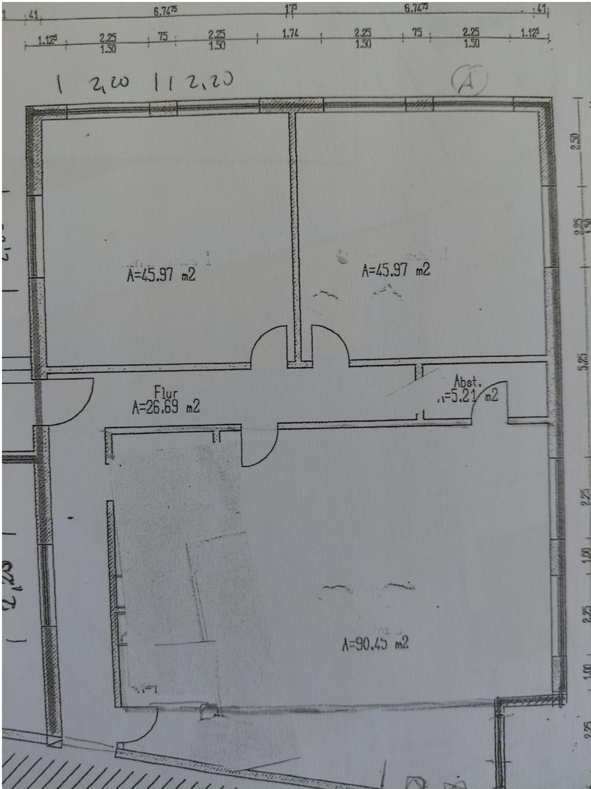
Grundriss 200 qm
