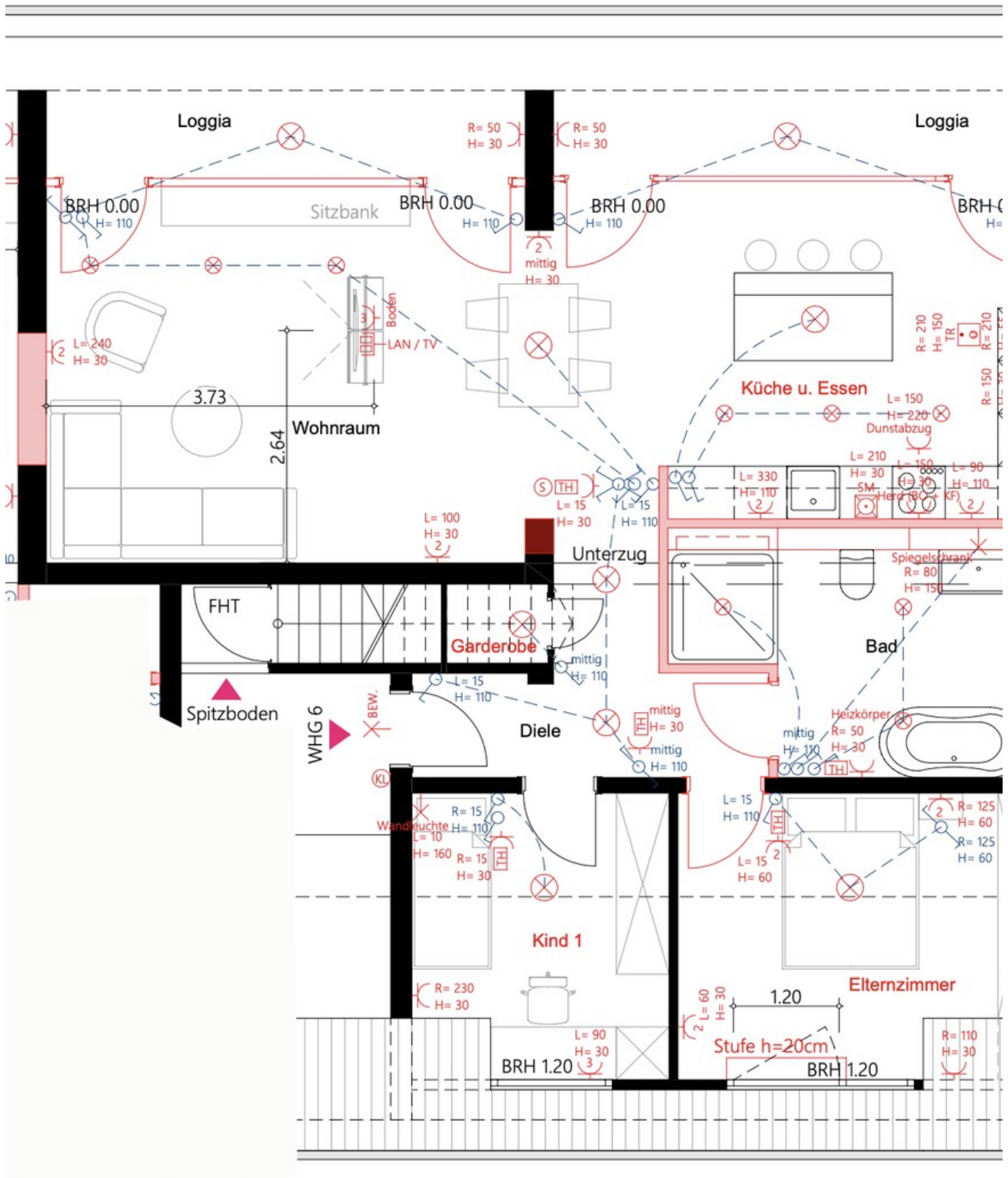
Whg 6 Grundriss und Elektro
