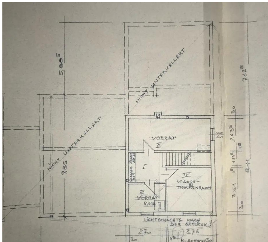
Grundriss Keller
