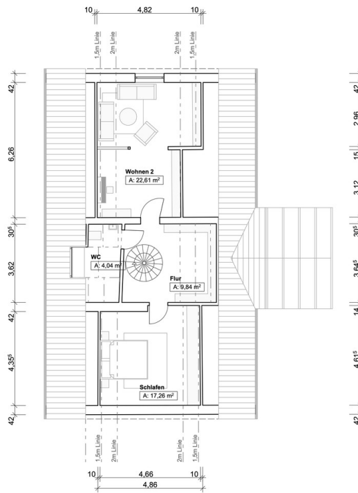
Grundriss Dachgeschoss
