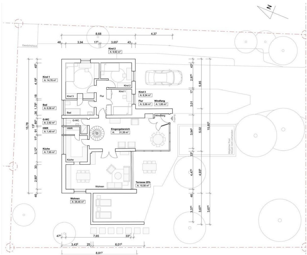
Grundriss Erdgeschoss
