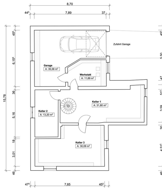
Grundriss Untergeschoss
