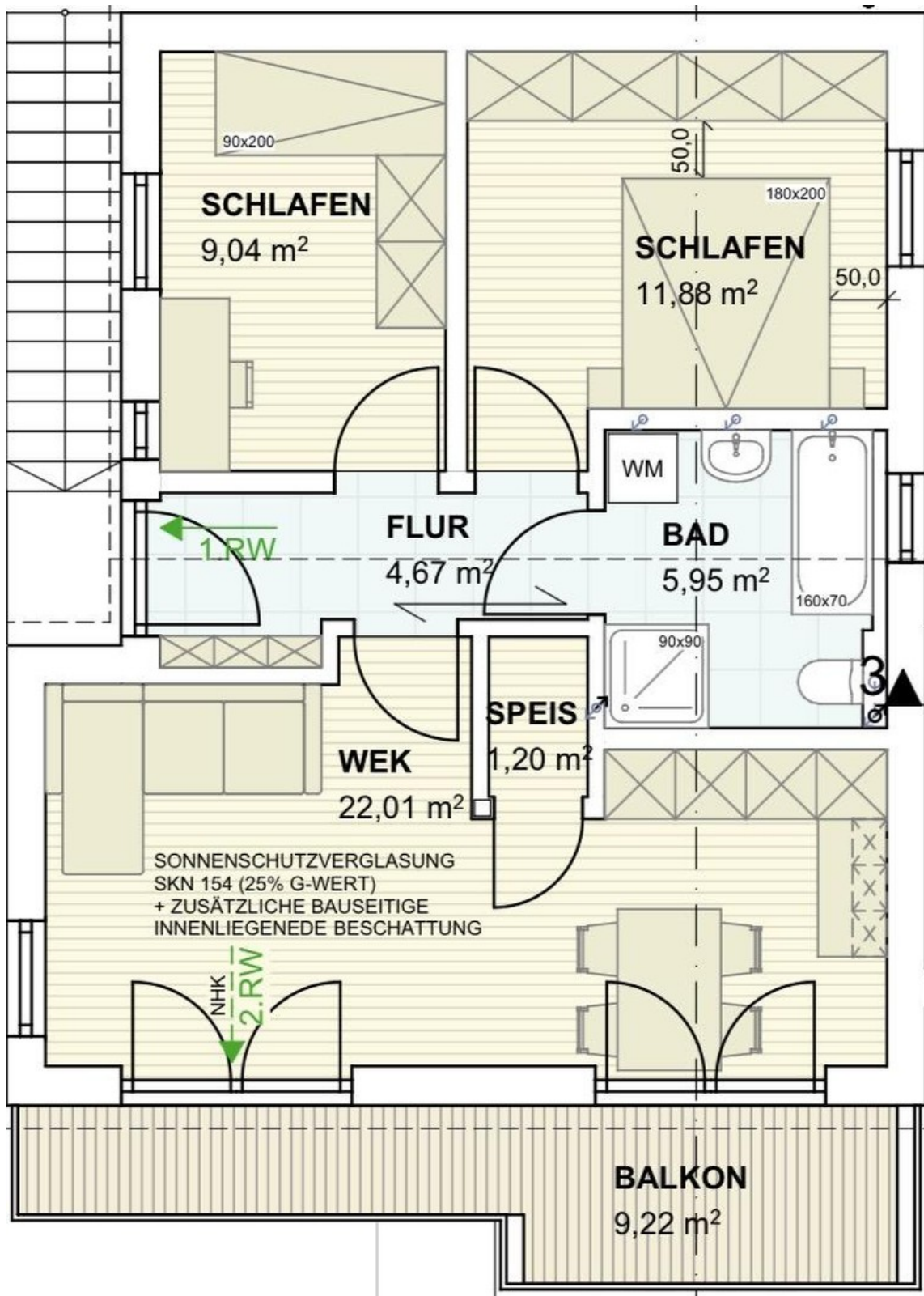
Grundriss Wohnung
