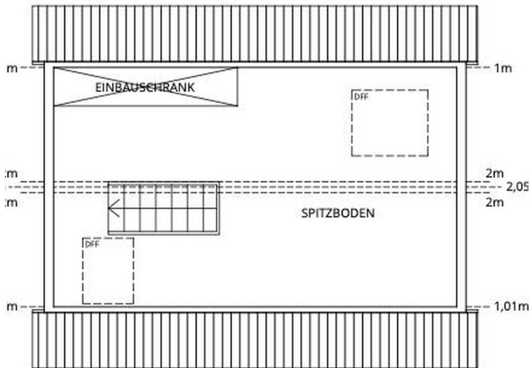
Dachgeschoss
