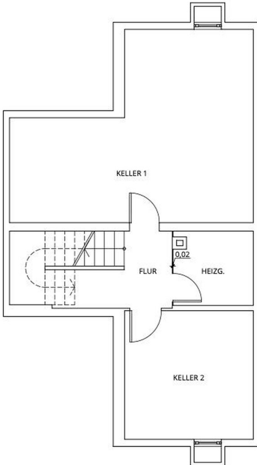
Keller
