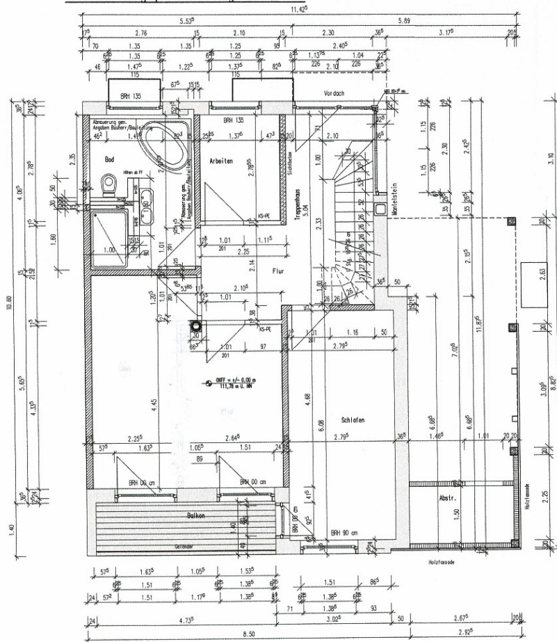
Ausführungsplan : Erdgeschoss
