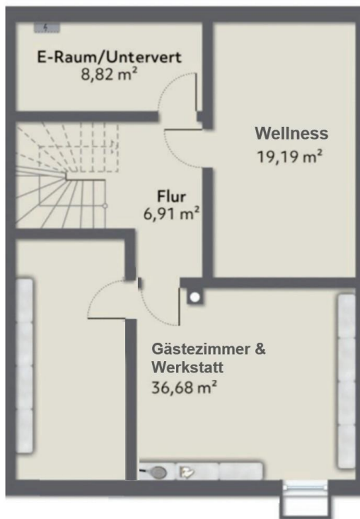
Grundriss KG
