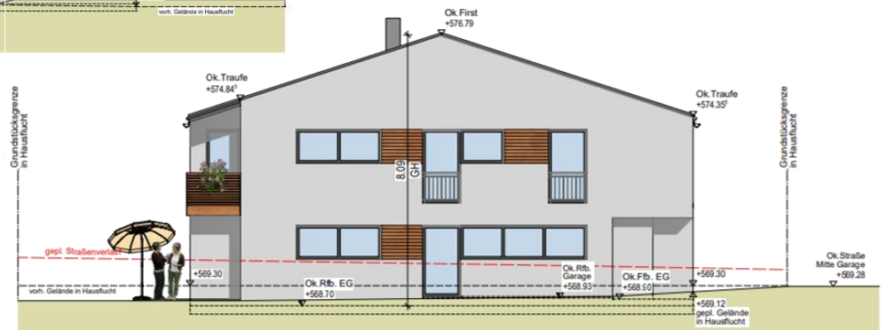
Osten
