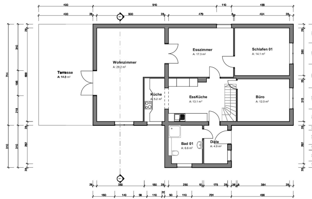
Erdgeschoss 1:100
