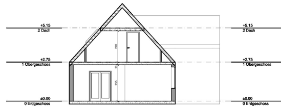
Schnitt 01 1:100
