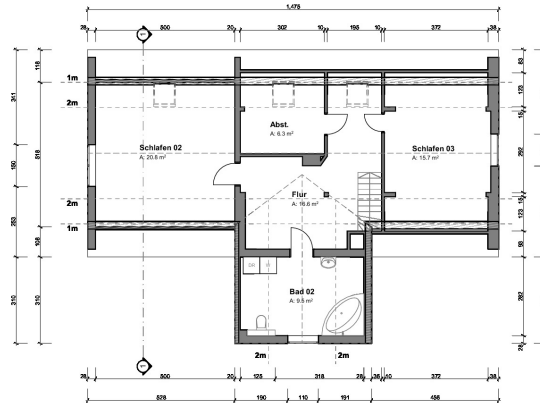
Obergeschoss 1:100
