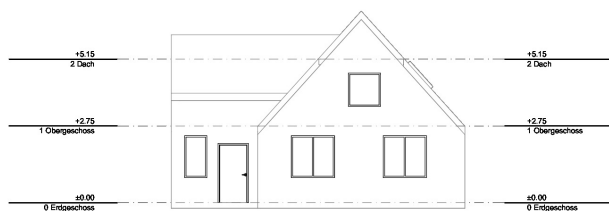
Ostansicht 1:100
