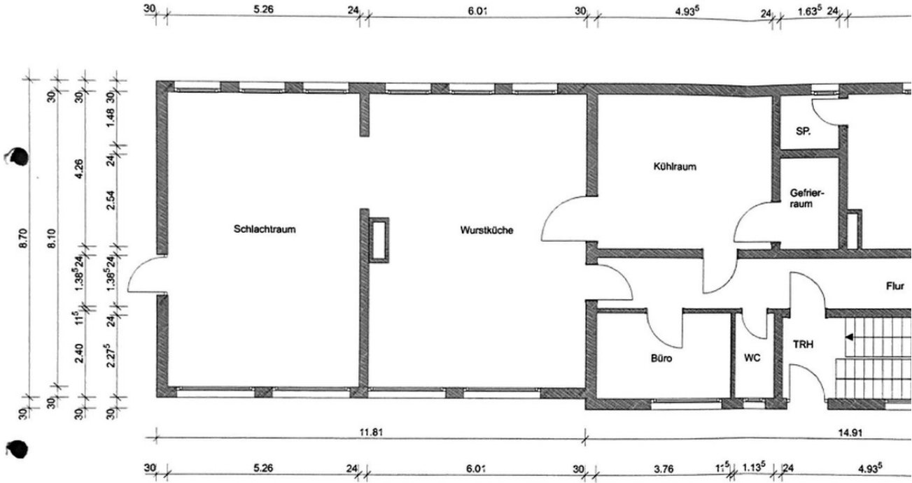
ERDGESCHOSS
