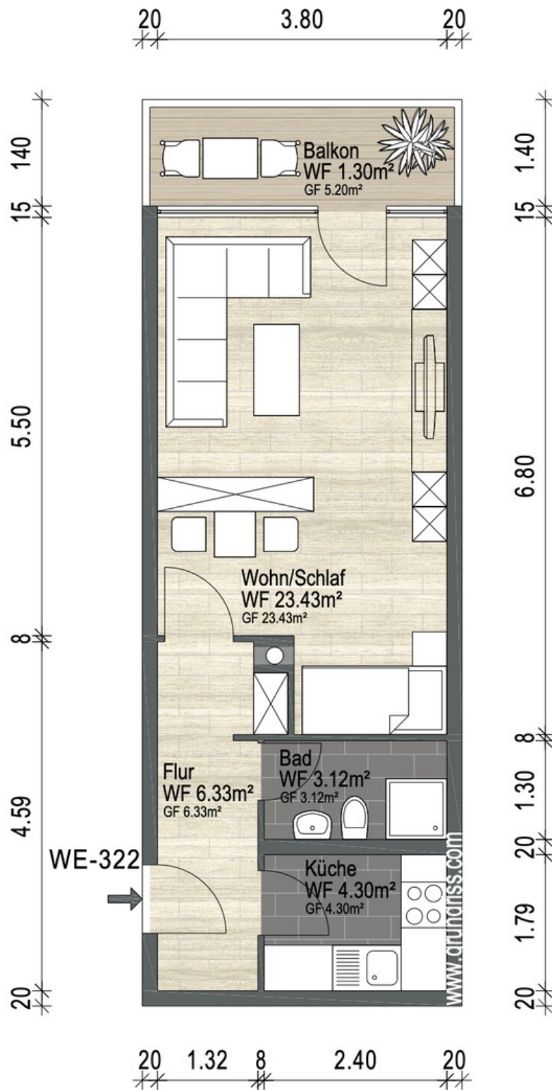
Grundriss
