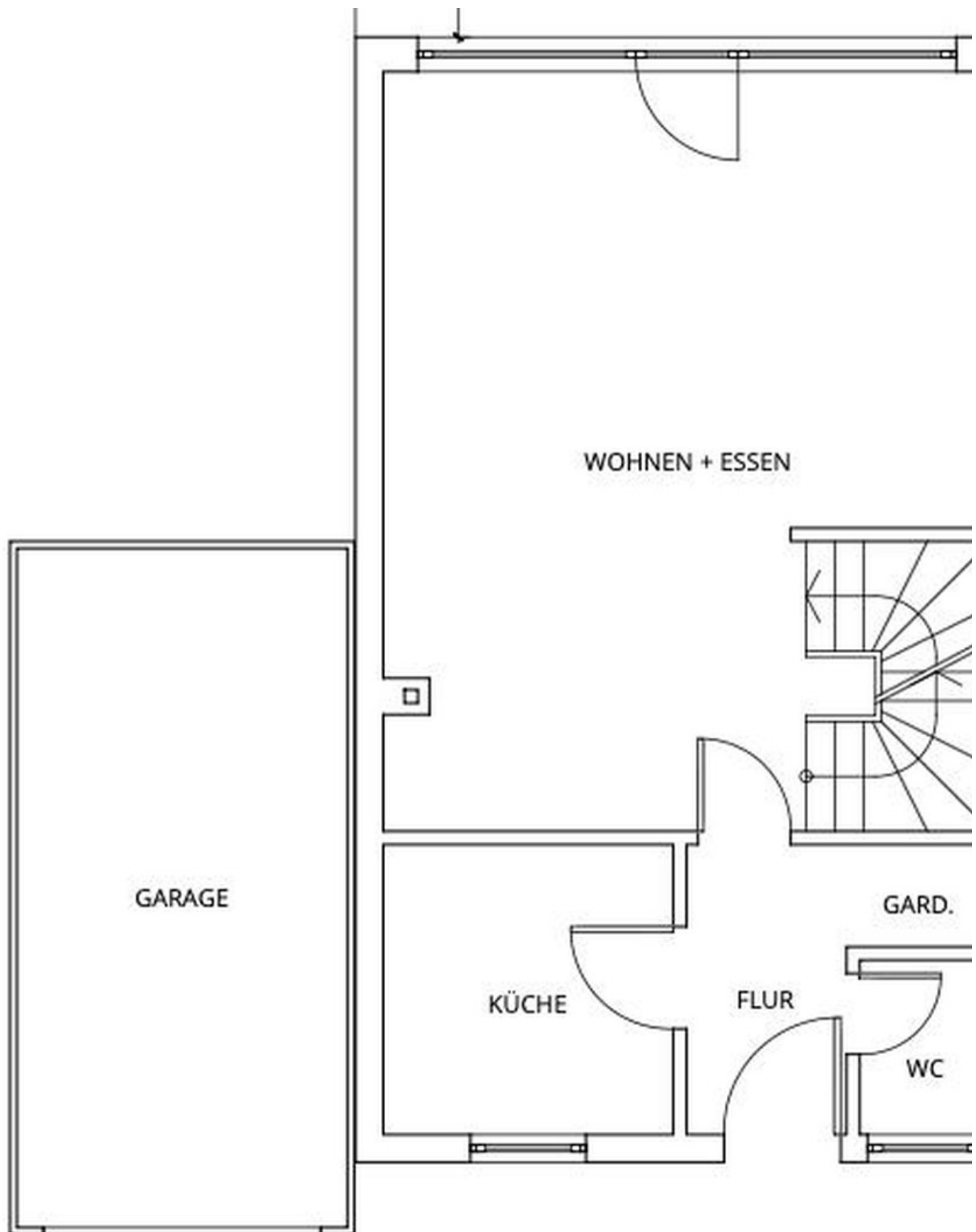
Erdgeschoss
