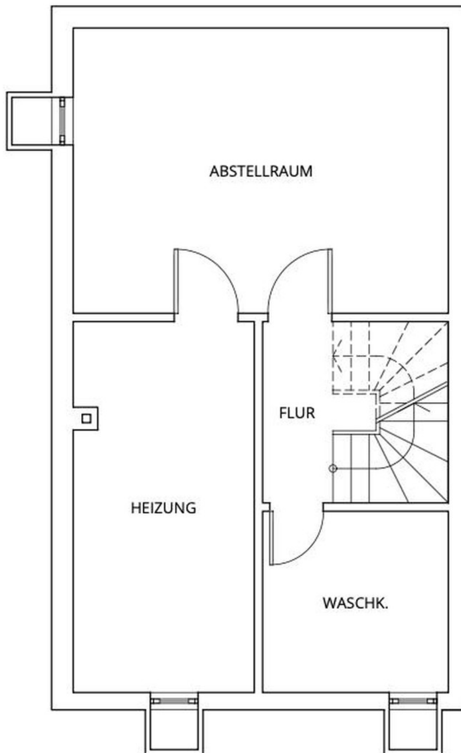
Keller
