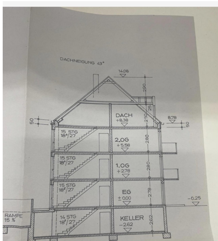
Grundriss Gesamthaus
