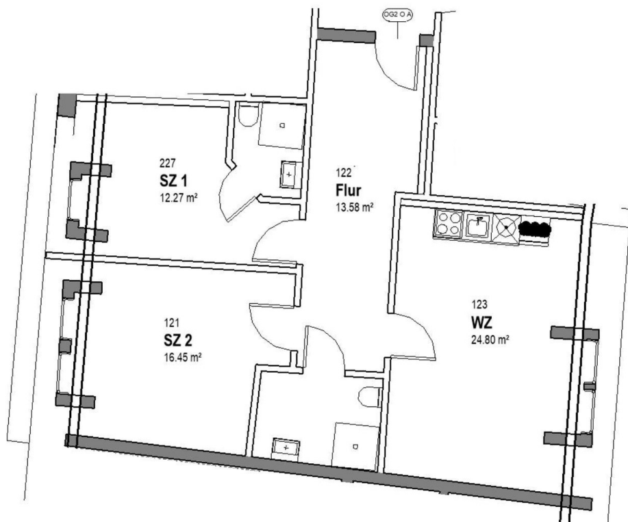
Grundriss
