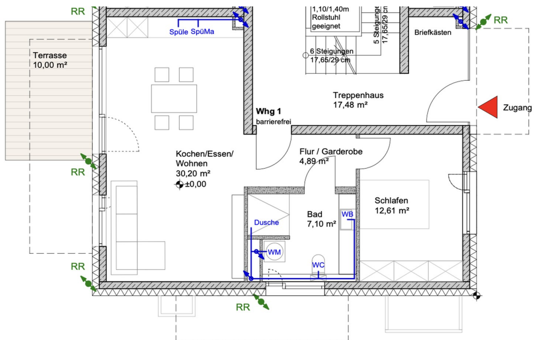
Grundriss EG
