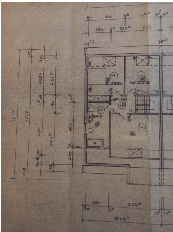
Lageplan Obergeschoss
