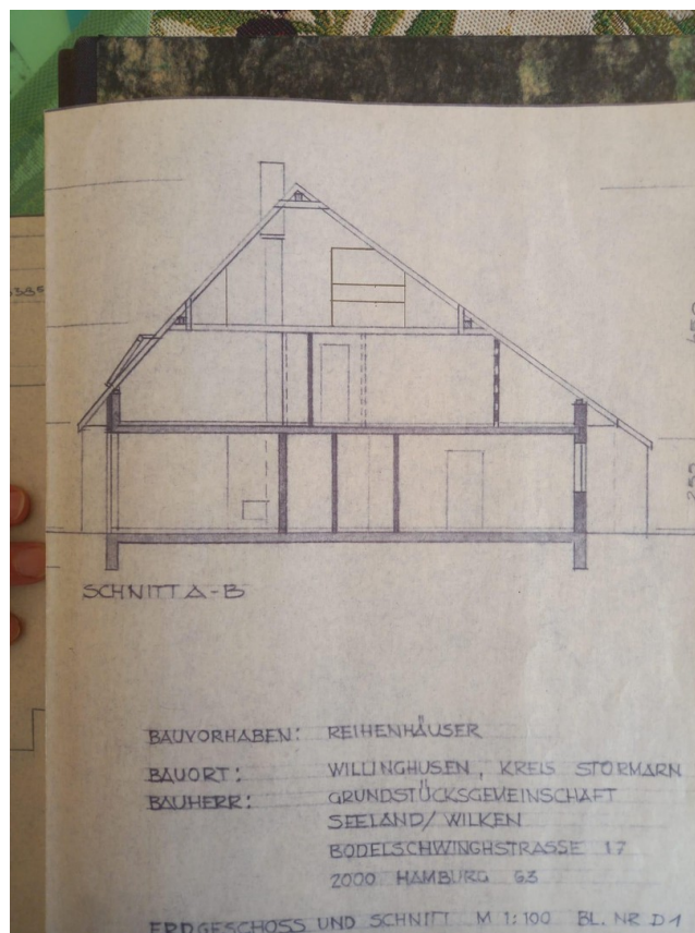
Schnittbild
