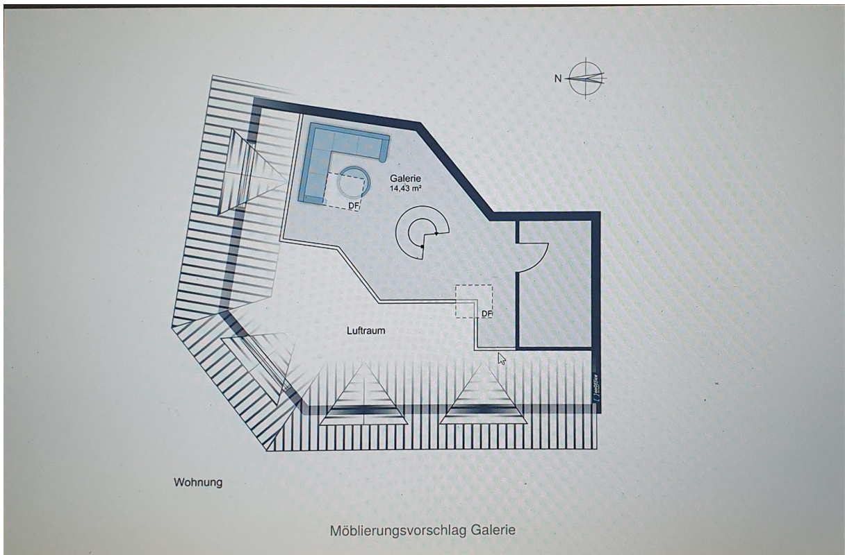
Grundriss Ebene 2
