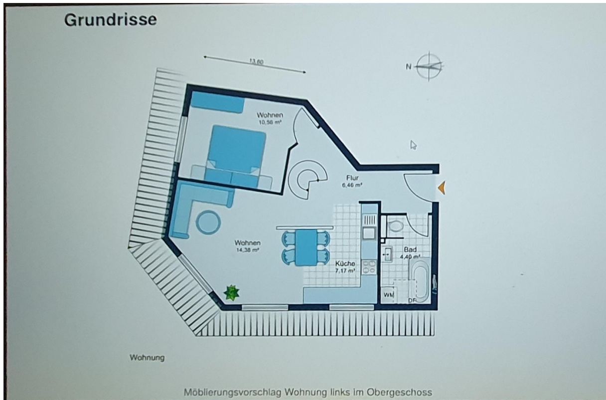
Grundriss Ebene 1
