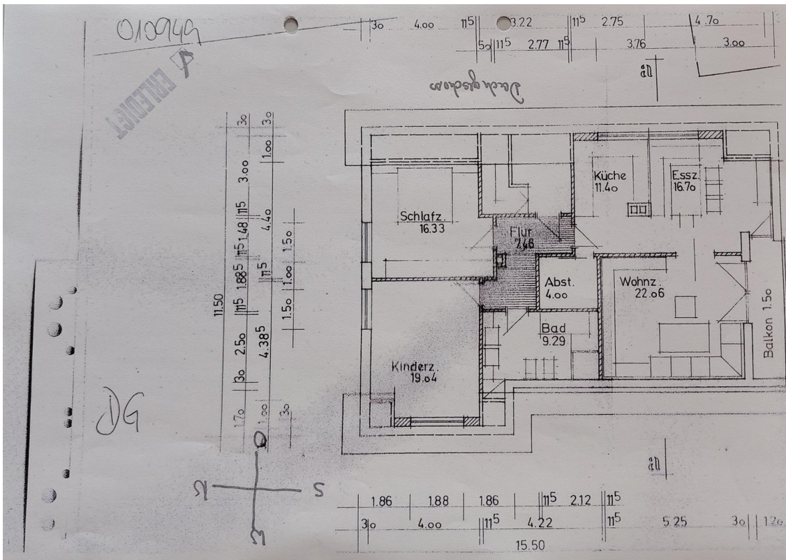
Grundriss Dachgeschoss
