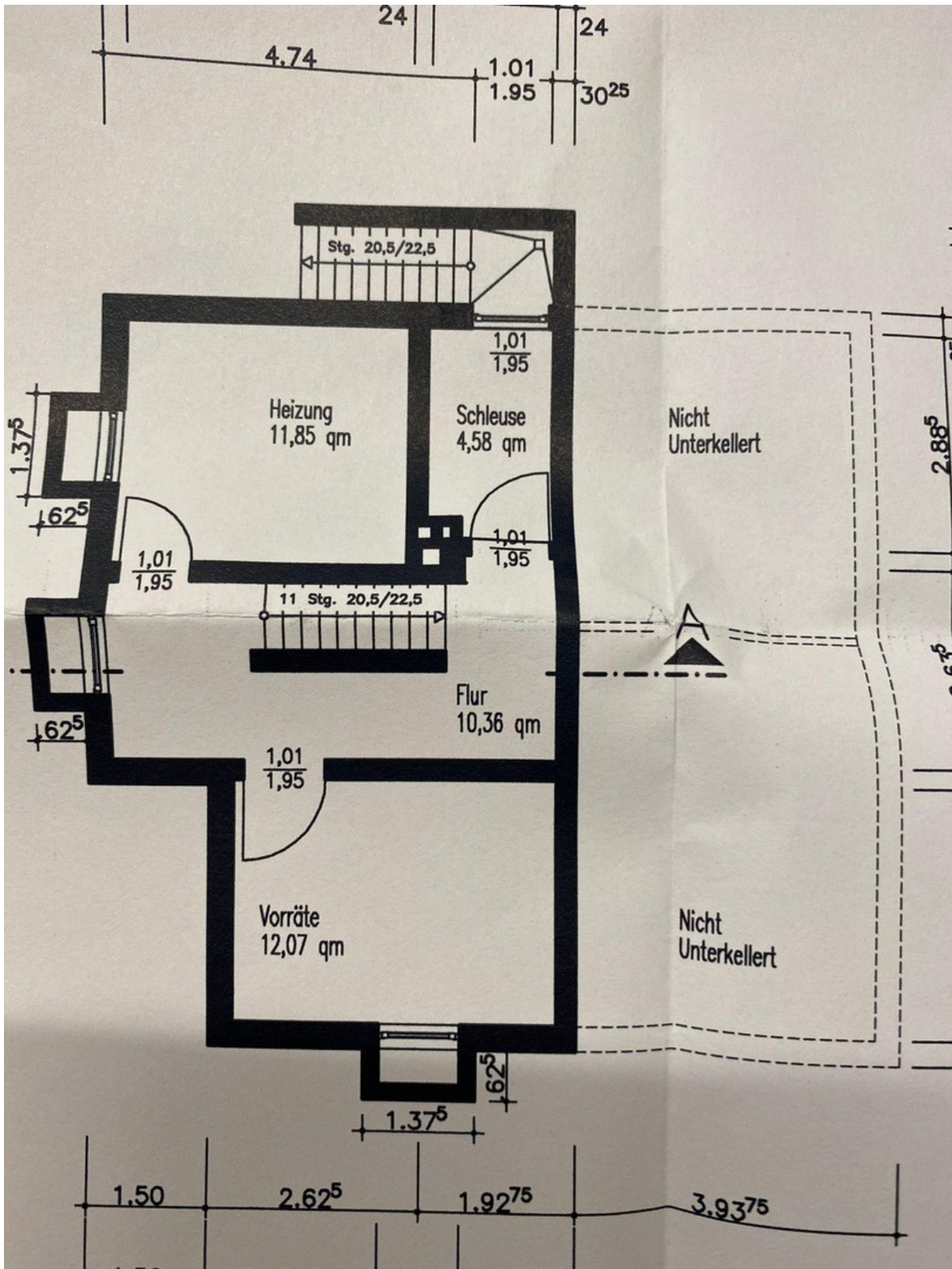
Grundriss Kellergeschoß
