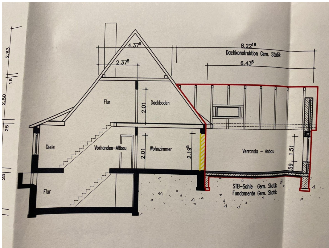
Schnitt UG - DG
