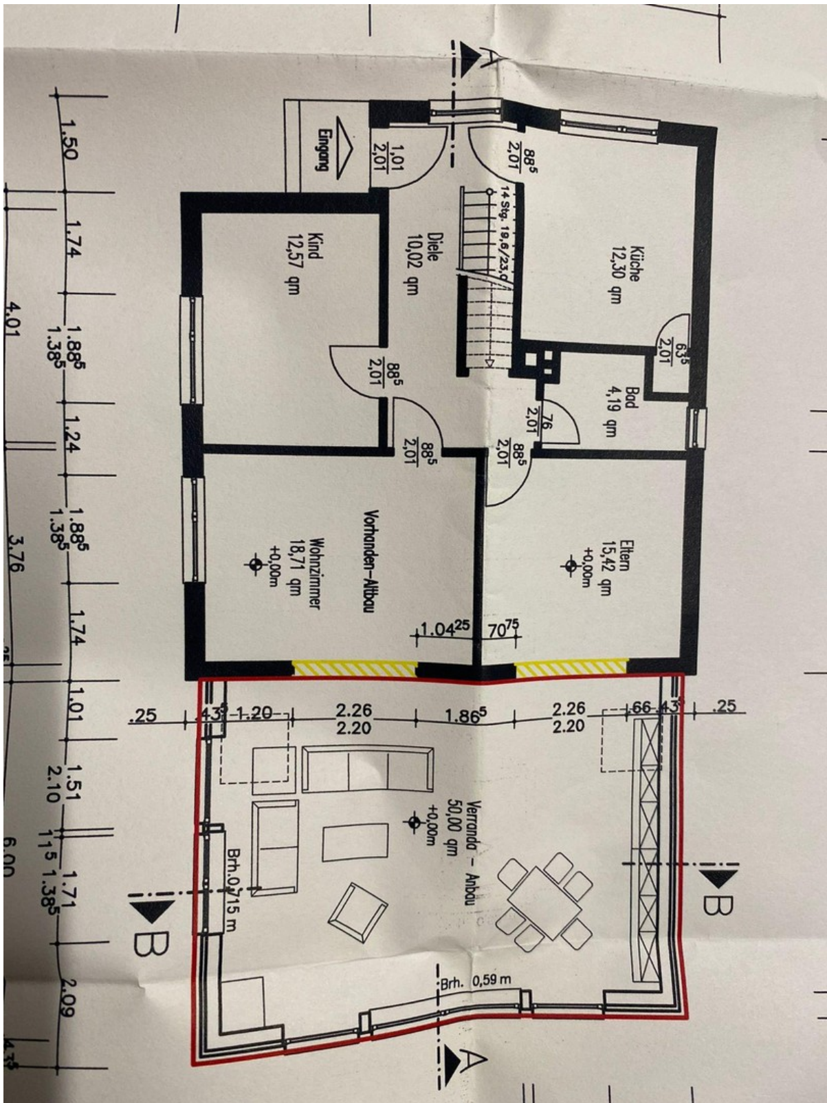
Grundriss Erdgeschoß
