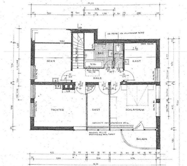
Obergeschoss
