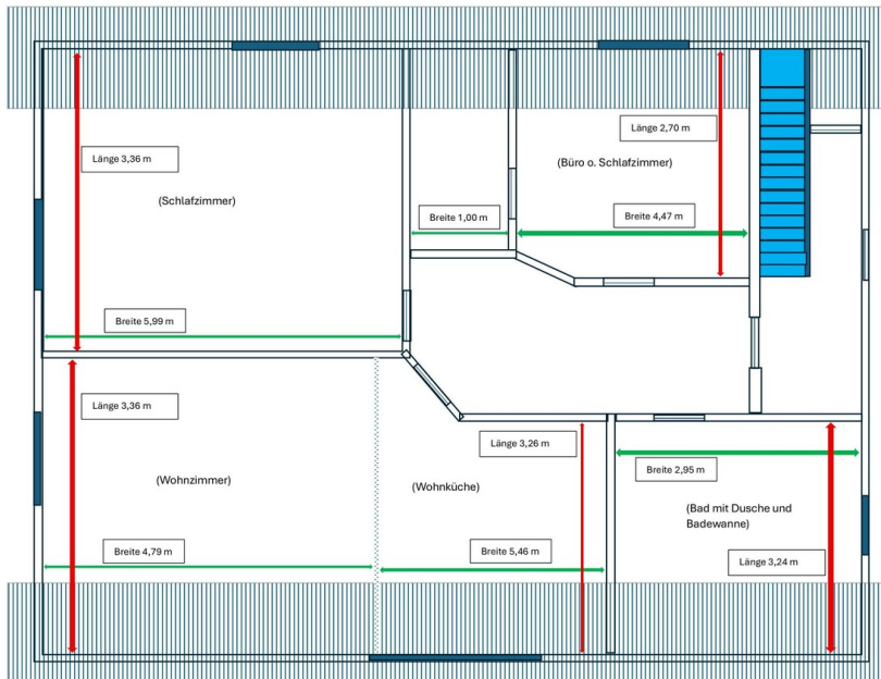
Grundriss Wohnhaus OG
