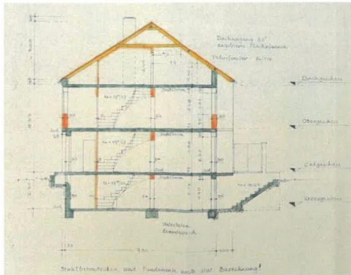
Schnitt - Reihenmittelhaus
