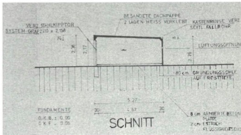
Schnitt - Garage
