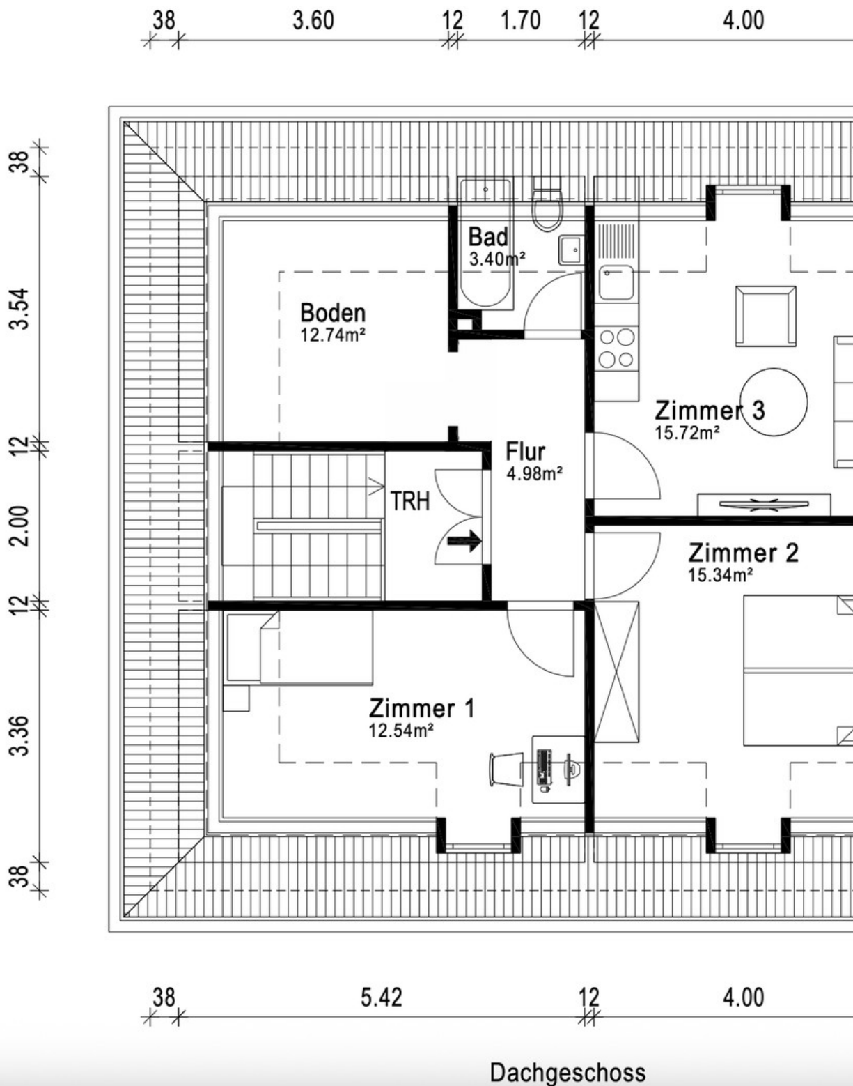
Grundriss Dachgeschoss
